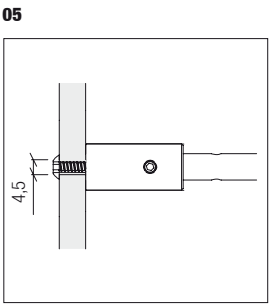
Montage sur acrylique Mounting onto acrylic glass
