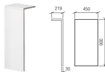
01 Bandeau frontal en dérivé de bois peint, avec profil circonférentiel en acier époxy noir
