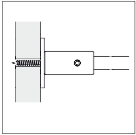
Montage auf Gipskarton/ Mauerwerk Mounting onto plasterboard/ brickwork
