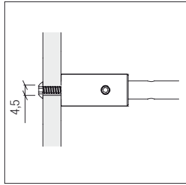
Montage auf Acrylglas Mounting onto acrylic glass
