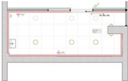
Planungsbeispiel Umbau: Planning example reconstruction:
