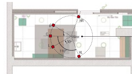
5.1 Lautsprecher System 5.1 speaker system
